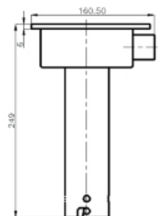
天井取り付けブラケット HAS1CLMDZE
