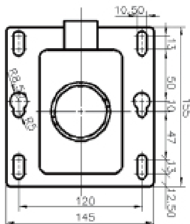
壁ブラケット HAS1WLMDZE
